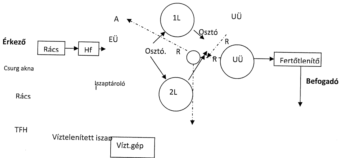
Újfehértói Szennyvíztisztító Telep Blokksémája
